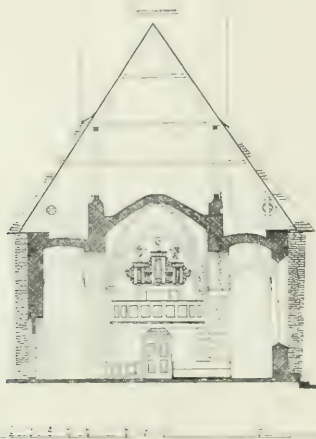
Fig. 25. Tvärsnitt av långhusets närmast tornet belägna travée visande orgel och dess laktare. Efter uppmätning av S. Curman o. A. Roland 1907, kompletterad av H. Sundberg 1927. Querschnitt durch das westlichste Transversal section of the nave com- Joch des Langschiffes, die Orgel und partiment nearest the tower, showing ihr Emporenzeigend the organ and its gallery.
